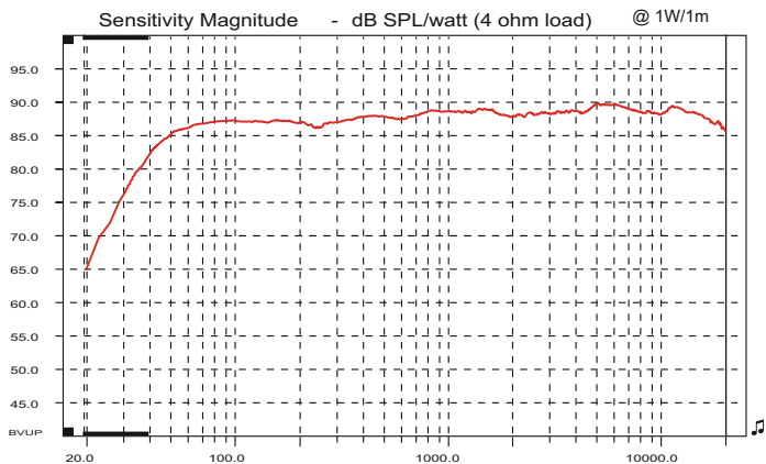
CURVA DI RISPOSTA DEL SISTEMA TRIO LA 6/10
